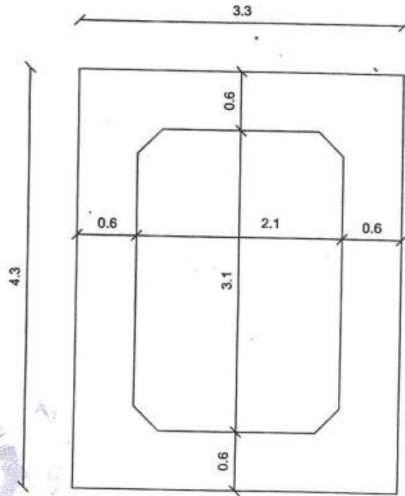
Plinth plan
