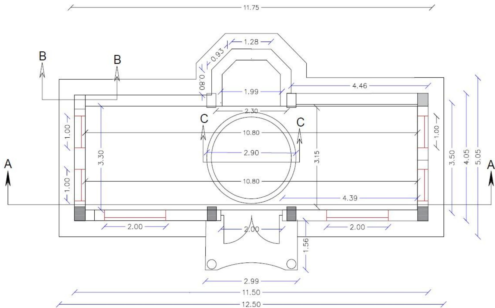
مسجد شريف نقشه
