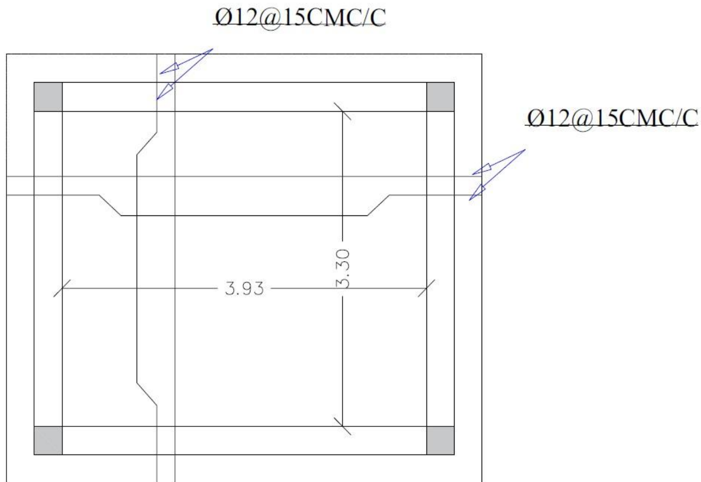
د تشناب سيخ پلان
